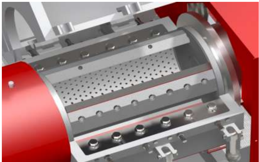
Ножи подвижные / не подвижные для роторной дробилки и агломератора
